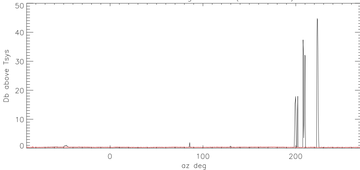
819.14 birdie strength vs az (rbw=21Khz)
