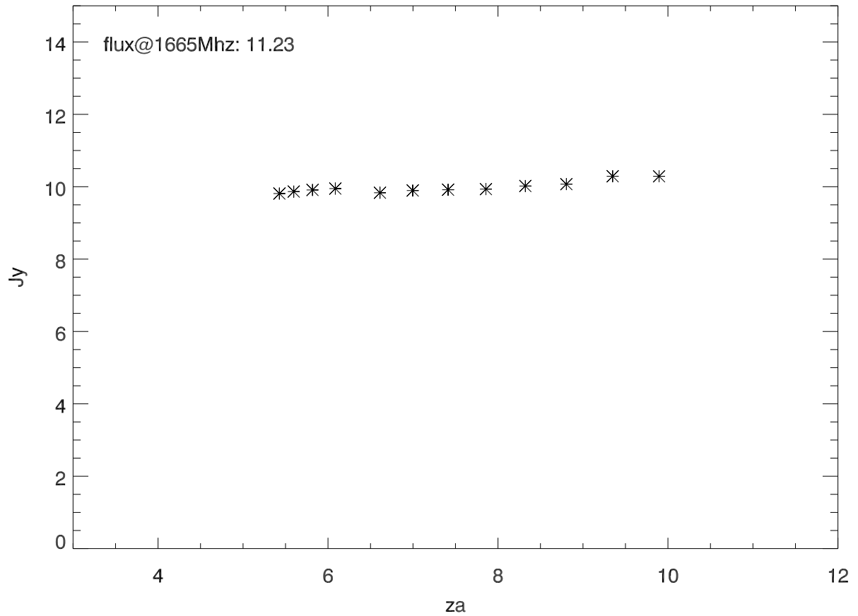
Sefd vs za
