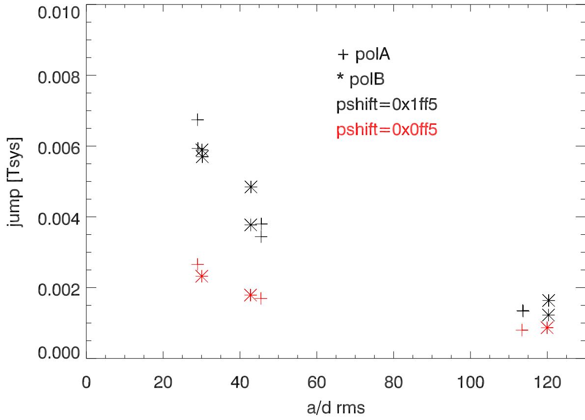
chan 2048 jump vs a/d rms
